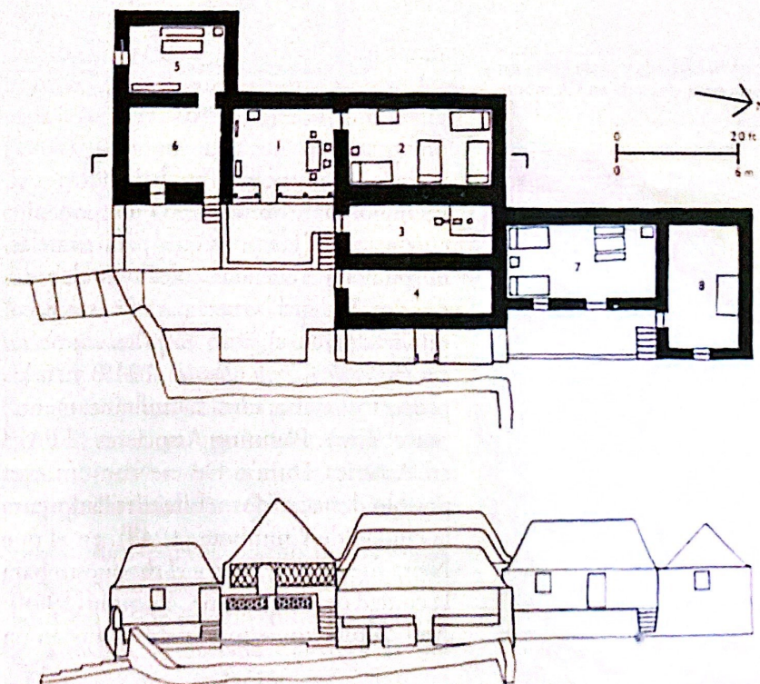
Figura 7. Planta baja y fachada de una casa en Congata.
