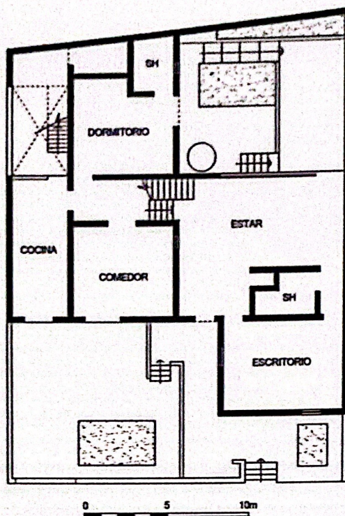
Figura 2. Casa Neira, planta baja del primer piso.
