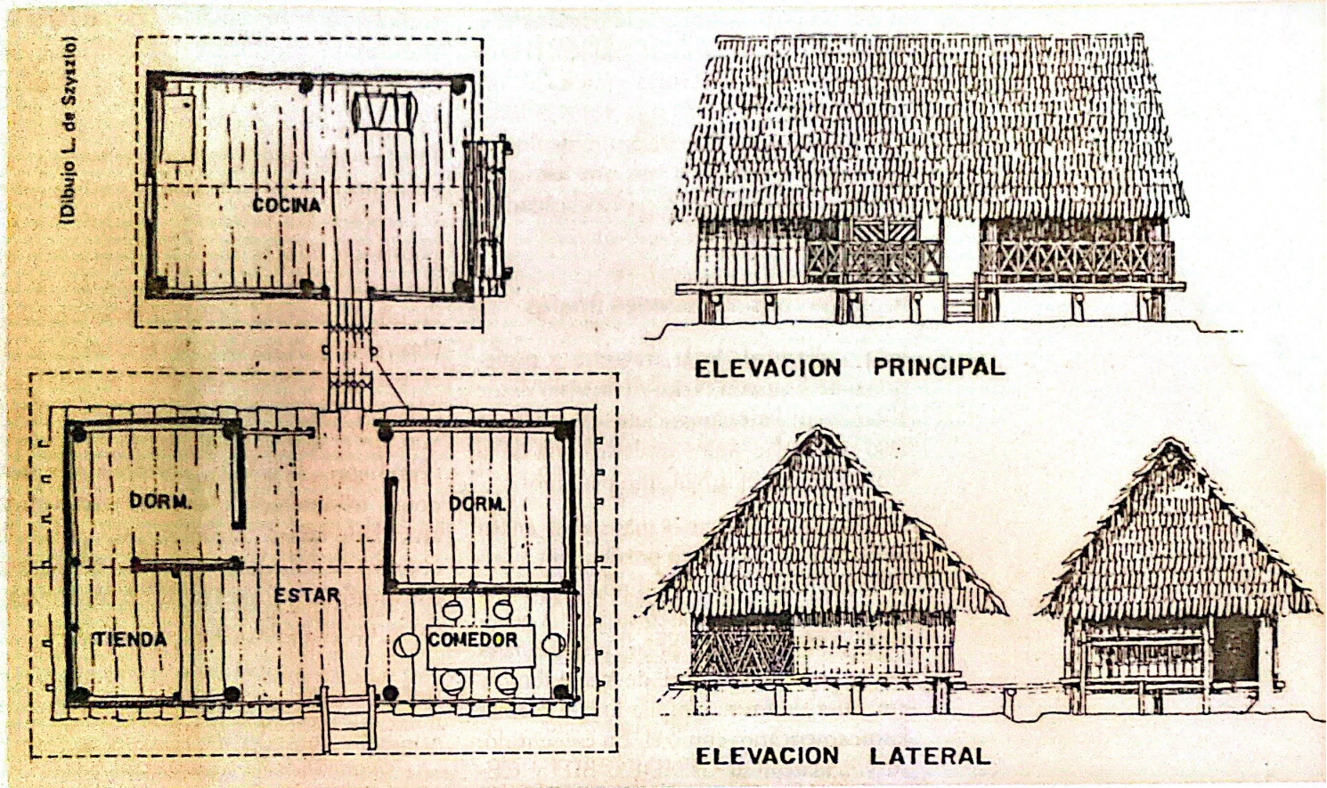
Figura 13. Vivienda piros. Planta y elevación del grupo familiar ete-ne en el asentamiento Miaría (Bajo Urubamba)
