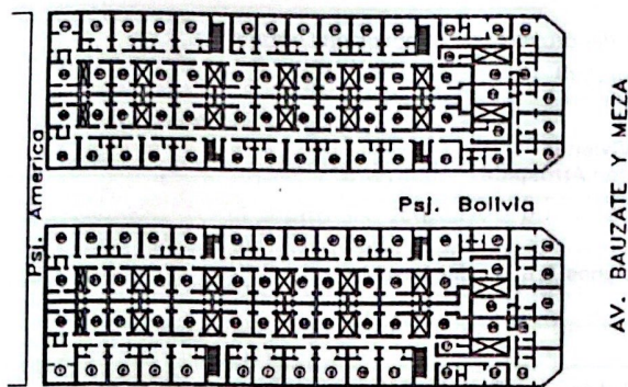
Figura 2. Planta típica de los 2 edificios intervenidos. Fuente. Patricia Iriarte, Roberto Lecca. 2011.
