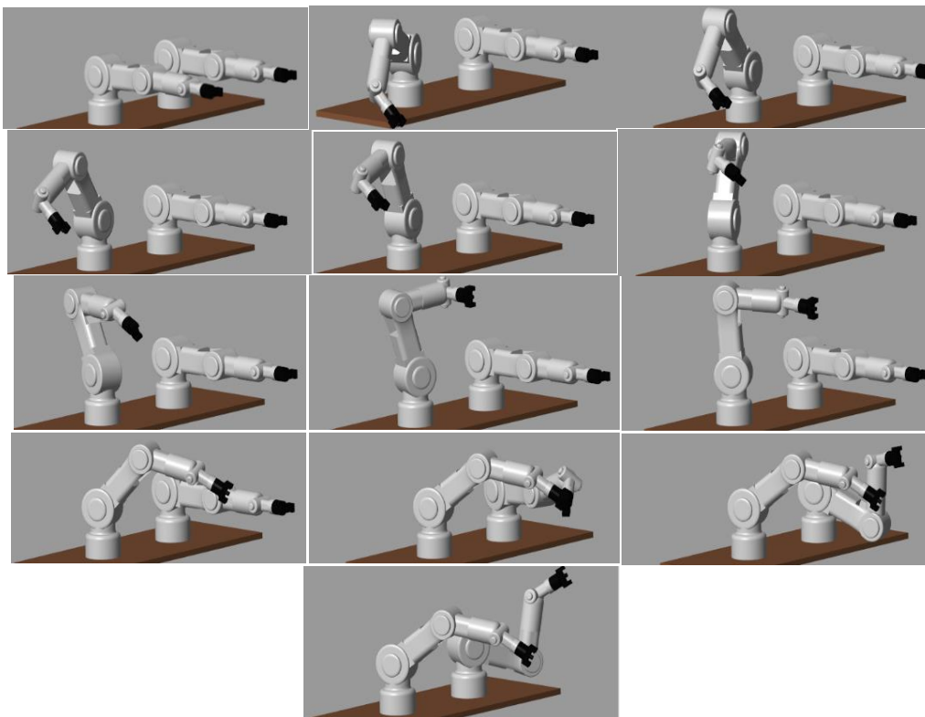
Fig. 8. Secuencia de movimientos de los robots 1 y 2 al simular el modelo de bloques de Simulink bajo las trayectorias propuestas.
