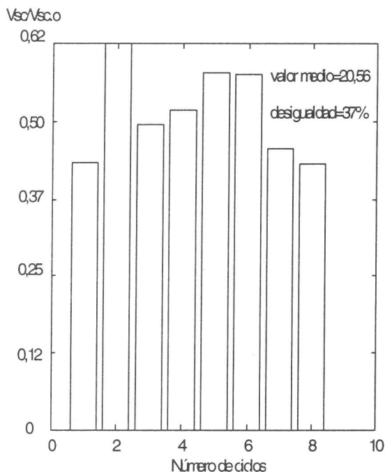
Fig. 9- Histograma del suministro cíclico, con RND, para n=300 rpm y h_{cremallera}=7 mm, V_{sc.o}=40 mm 3 .
