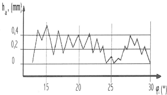
Fig. 2- La característica del levantamiento de la aguja del inyector de un motor diesel (4 tiempos, 6 cilindros, D \times S = 250 \times 340 mm) para bajas velocidades de rotación /4/.
