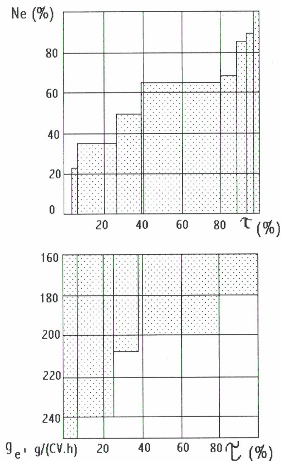
Fig. 1- Variación de la carga ( N_e ) y de la economía de combustible ( g_e ) de un motor diesel de tractor durante su funcionamiento ( \tau : tiempo) /2/.
