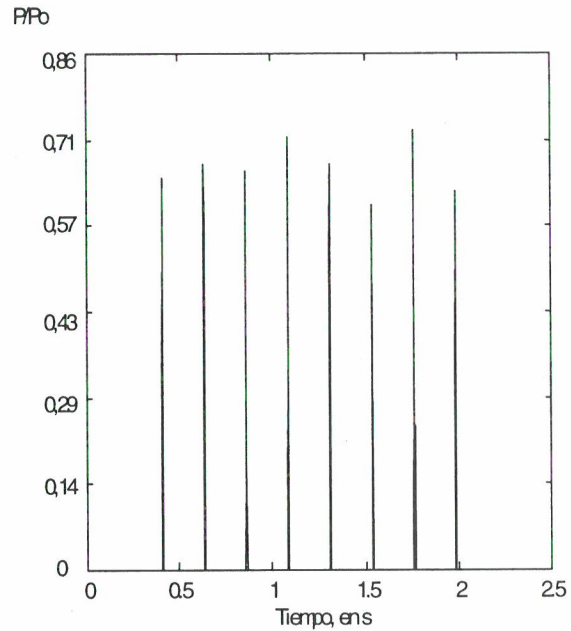
Fig. 7- Oscilograma de presión, con RND, para n=300 rpm y h_{cremallera}=7 mm, P_o=40 MPa.
