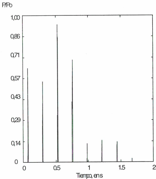
Fig. 6- Oscilograma de presión, sin RND, para n=300 rpm y h_{cremallera}=7 mm, P_o=40 MPa
