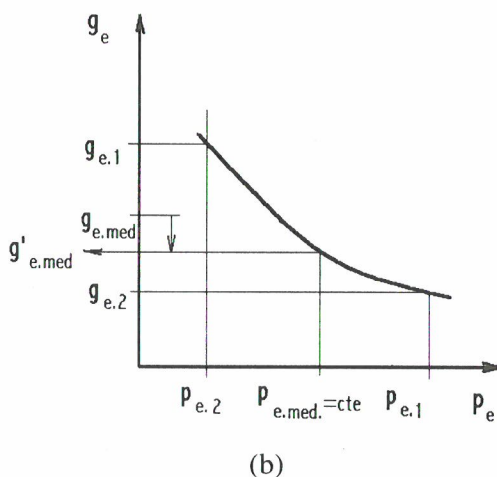
Fig. 4- Influencia de la estabilidad de la velocidad de rotación del cigüeñal ( n ) (curva a) y de la carga ( p_e ) (curva b) en el consumo específico de combustible ( g_e ).
