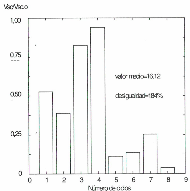
Fig. 8- Histograma del suministro cíclico, sin RND, para n=300 rpm y h_{cremallera}=7 mm, V_{sc.o}=40 mm 3 .
