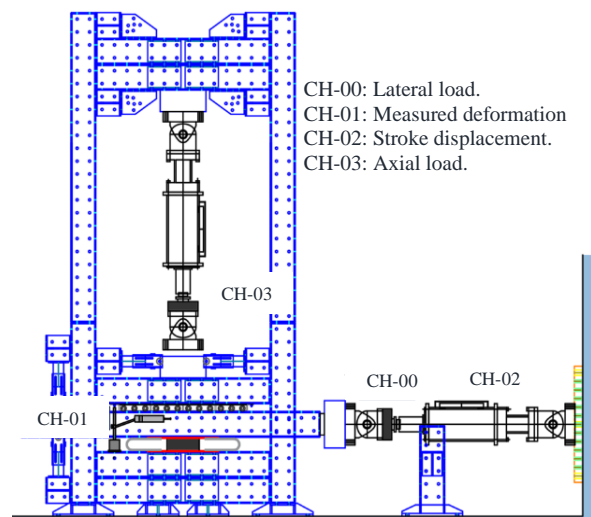
Fig. 8. PSD Test Setup [15].
