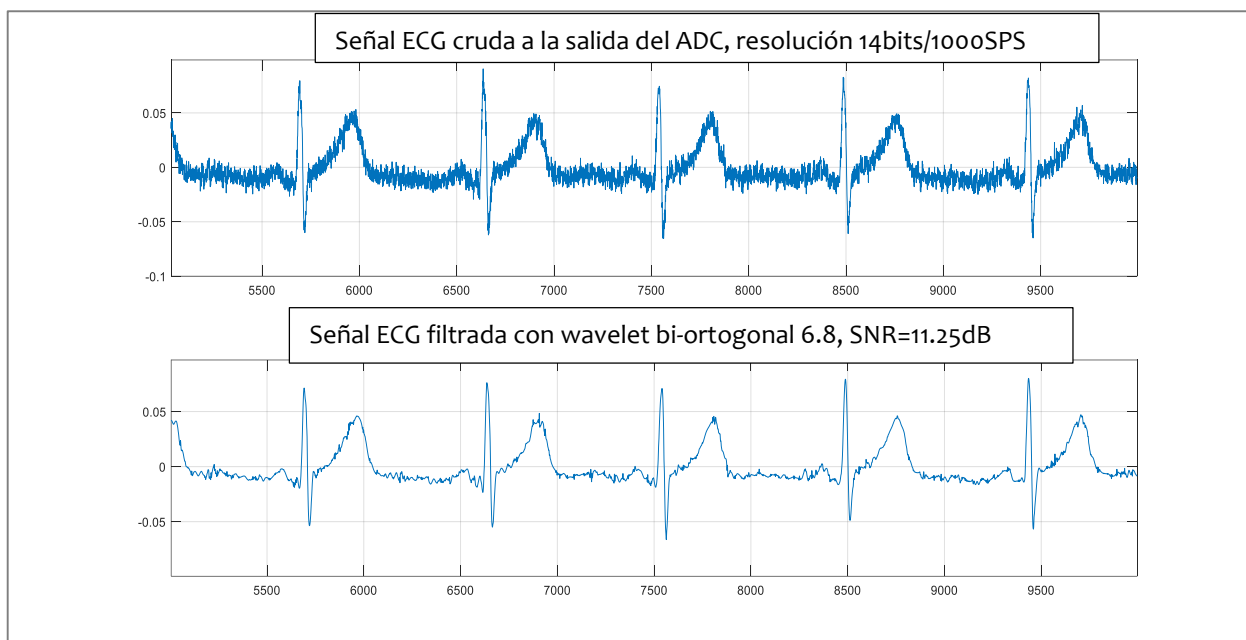
Fig. 3. Señal ECG cruda (zona superior) y señal ECG filtrada (zona inferior), USB-6009 National Instruments
