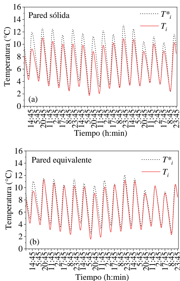
Fig. 9. Temperatura interior medida ( T_i ) y simulada ( T^*_i ) del 4 al 18 de junio de 2021, (a) para sólida y (b) pared equivalente.
