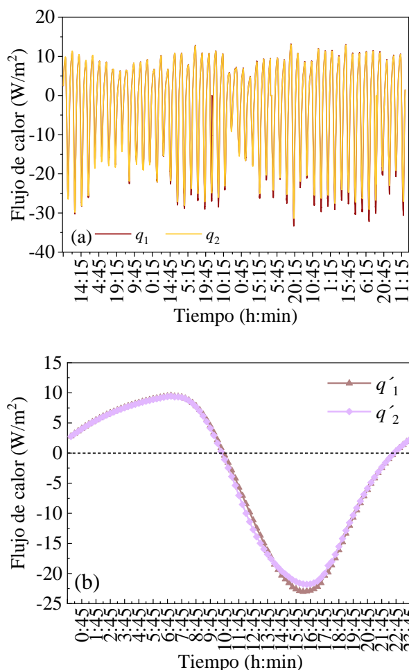
Fig. 8. Flujos de calor medidos en el lado interior de la pared de ensayo, (a) medidas diarias ( q_1 y q_2 ) y (b) promedio horario diario ( q'_1 y q'_2 ).
