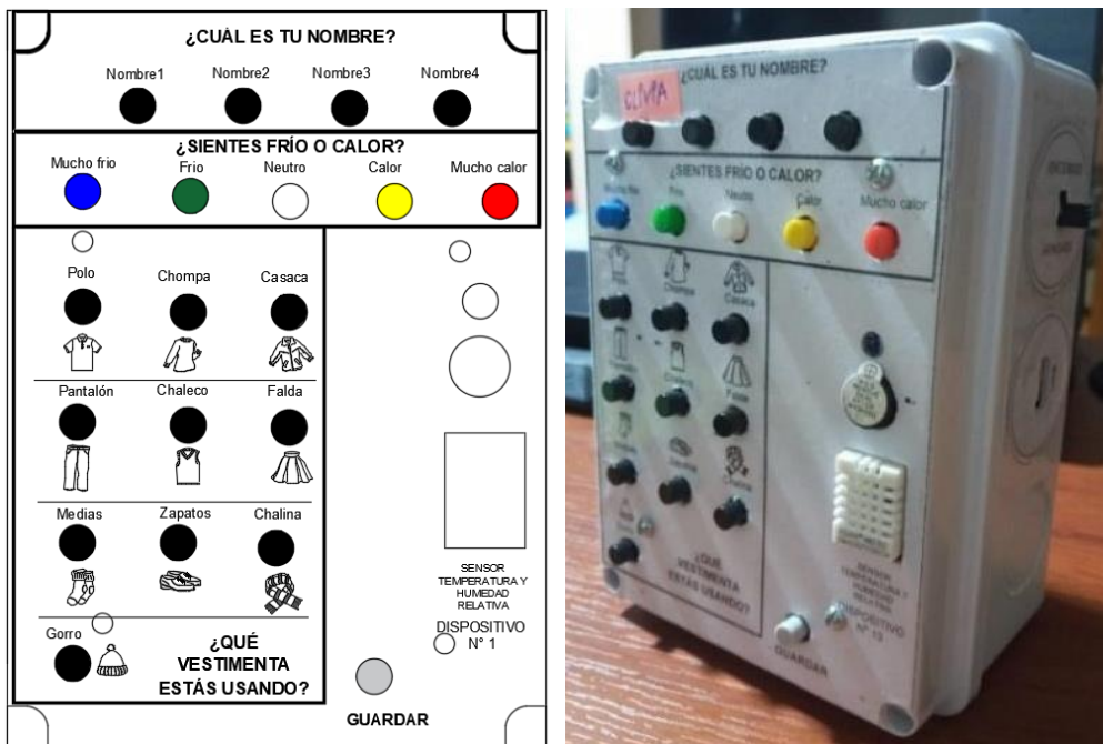
Figura 3. Esquema del dispositivo TSVR.
