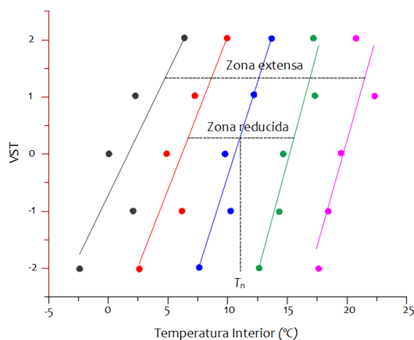
Figura 4. Valores promedio de la temperatura interior del total de datos.
