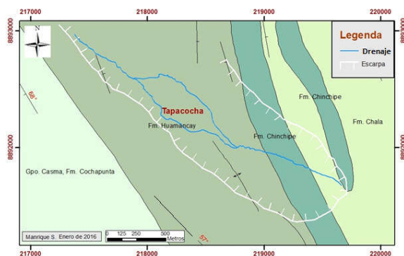
Figura 3. Plano litológico de Tapacocha.
