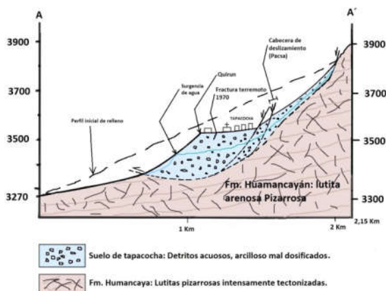
Figura 10. Sección geodinámica interpretativa de Tapacocha.
