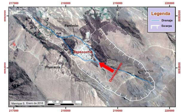
Figura 8. Interpretación geomorfológica de Tapacocha y alrededores.
