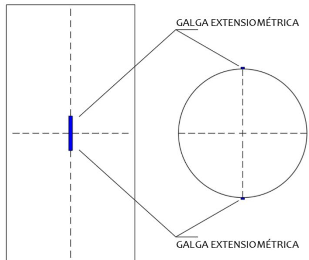
Fig. 4. Ubicación de las galgas extensiométricas en los especímenes de ensayo.
