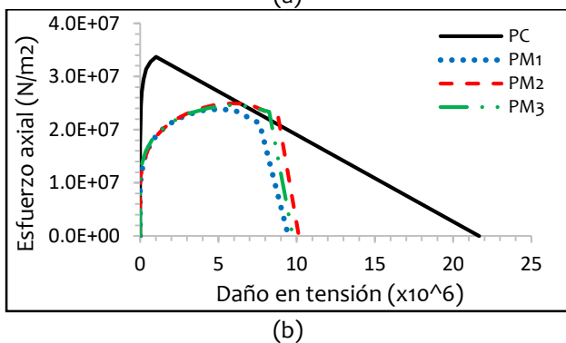
Fig. 10. Curvas daño-esfuerzo axial: a) daño en compresión, b) daño en tensión
