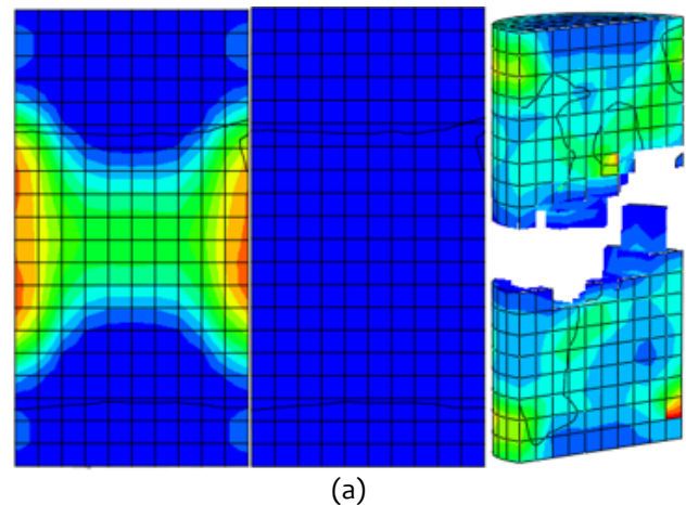
Fig. 9. Daño y subsecuente falla de los especímenes convencionales (a) y especímenes modificados (b)
