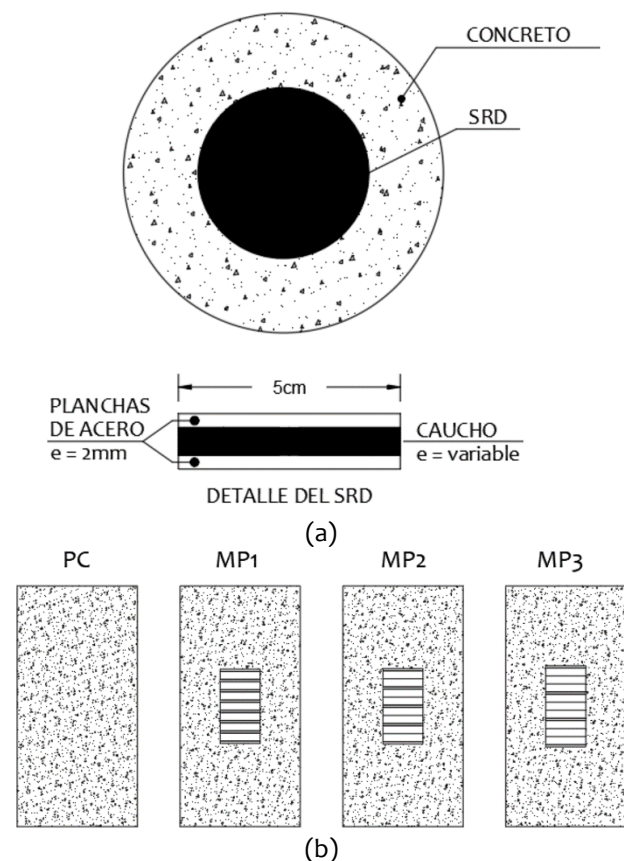
Fig. 1. Estructura y ubicación del SRD en las probetas de concreto (a) y configuración de cada espécimen de ensayo (b).
