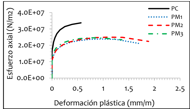
Fig. 8. Curvas esfuerzo-deformación plástica
